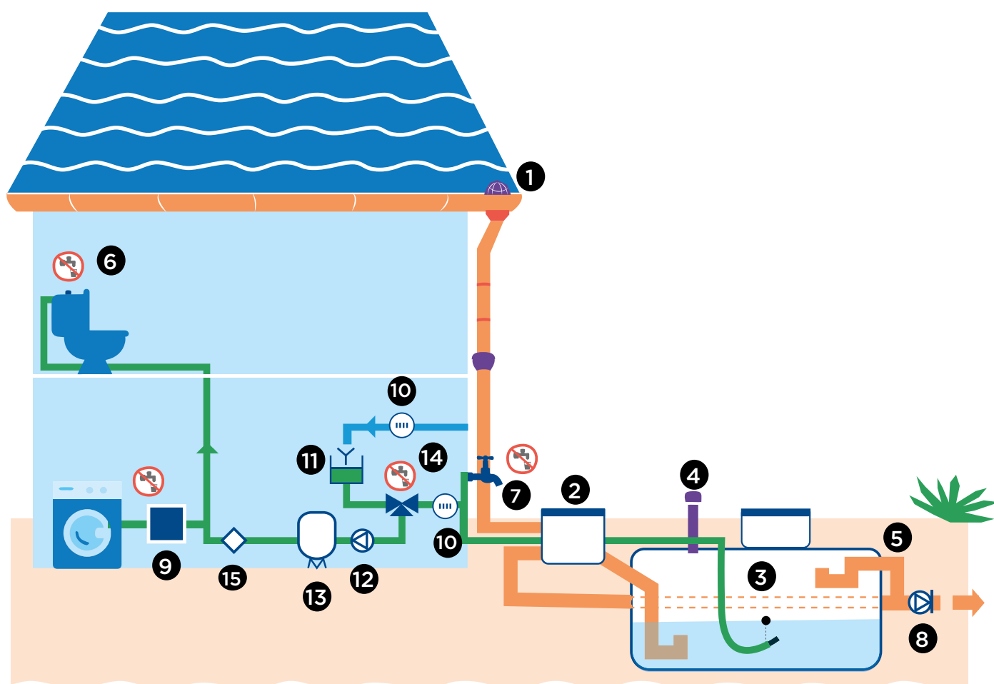
Installation d'une cuve enterrée pour un usage intérieur en logement individuel
