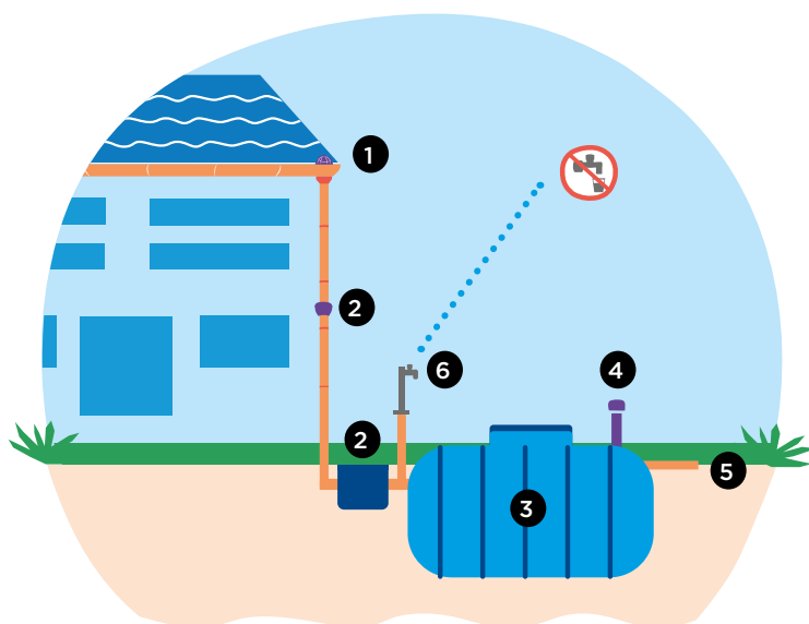
Installation d'une cuve enterrée
